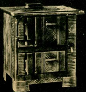
CF-13.567. CUISINIÈRE B. H. V. 52, tout en fonte émaillée gris ou castor, barre avant, à bain-marie, à retour de flammes, grand four chauffé sur 5 faces, foyer mixte bois et charbon. Longueur 0 m 75. 825.»
