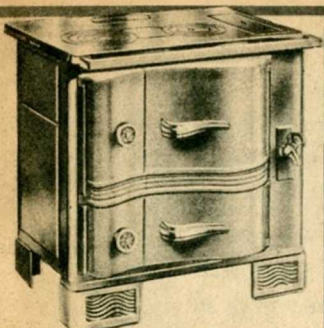
CF-13.559. CUISINIÈRE B. H. V. "Fedra" tout fonte, émaillée gris ou castor, barre avant, bain-marie, foyer charbon, départ de fumée dessus ou derrière, accessoires chromés. Longueur 0 m 65..... 689.»
